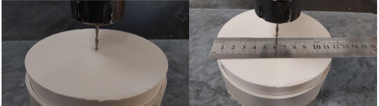
Şekil 8. CNC router makinesine alçı kalıpların sıfırlama işlemi.
